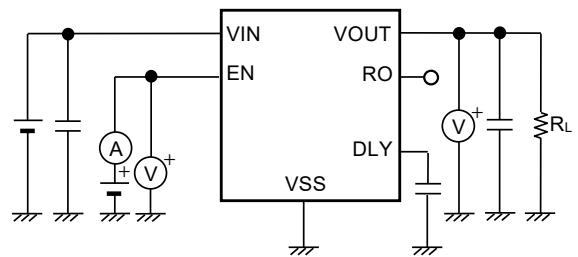
图9 测定电路4
