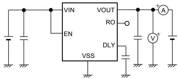
图7 测定电路2
