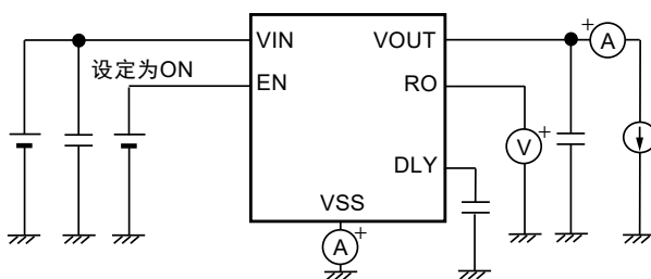
图12 测定电路7
