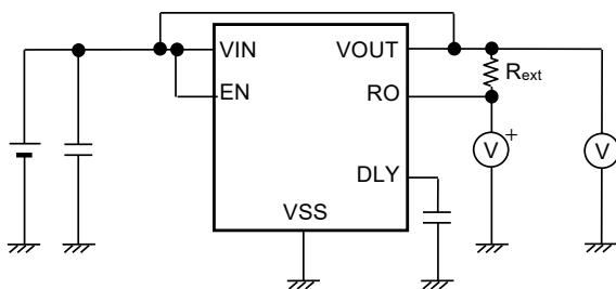
图10 测定电路5
