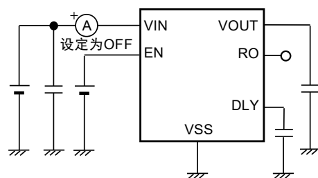
图13 测定电路8
