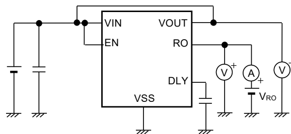
图11 测定电路6
